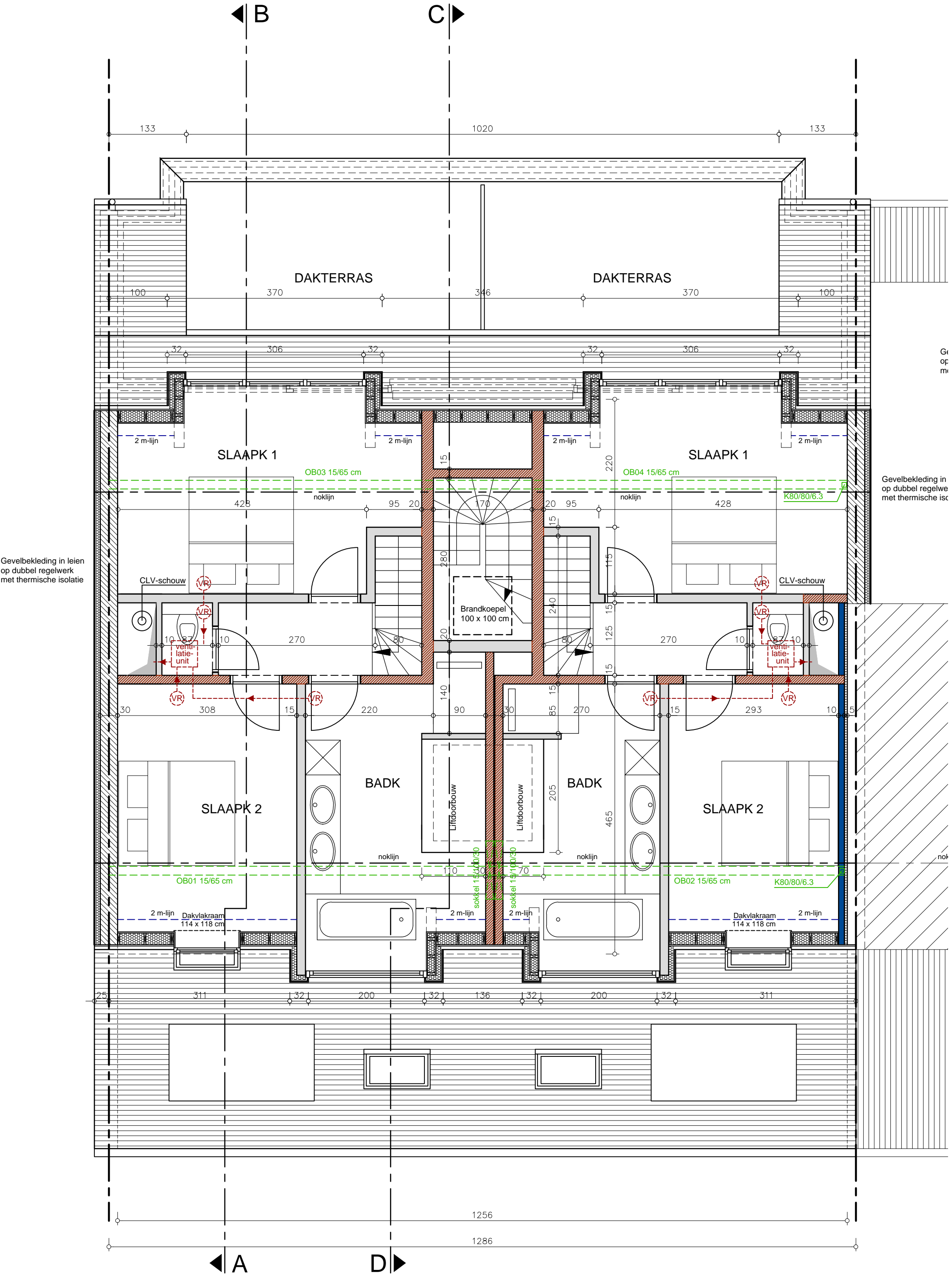
GRONDPLAN DUPLEXVERDIEP
